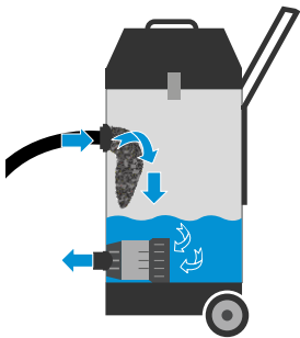
Funktionsprinzip
